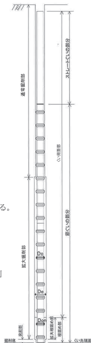
図-1-1 基礎ぐい設置概要図
