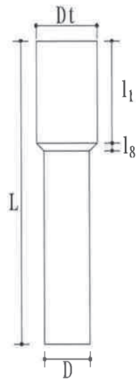
図-1-7 拡頭ぐい
